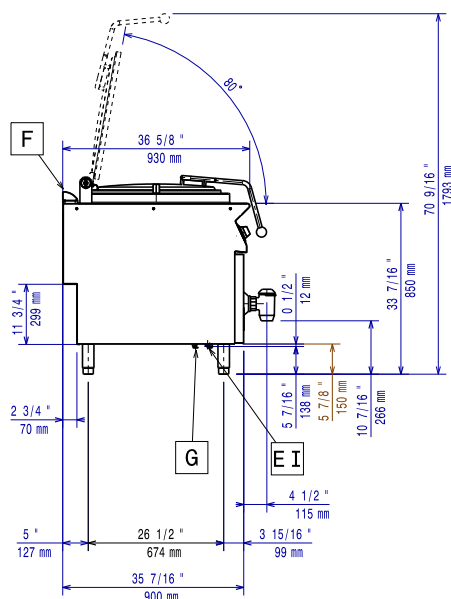
Zij aanzicht
